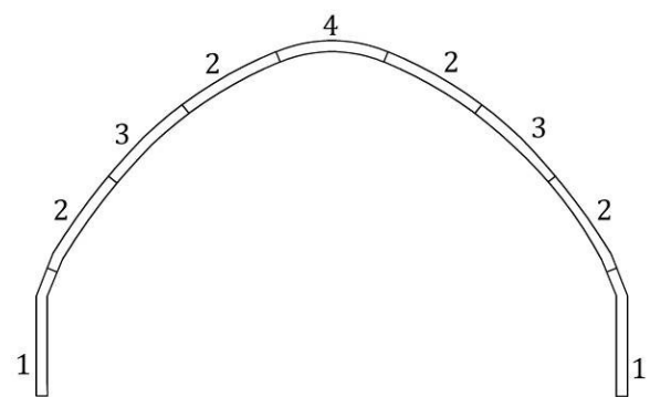
Etukaari ovenkarmilla
