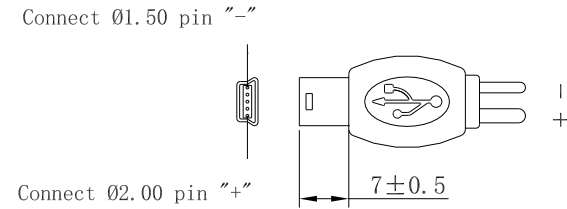
7. Mini USB-B 5 pin I type.
