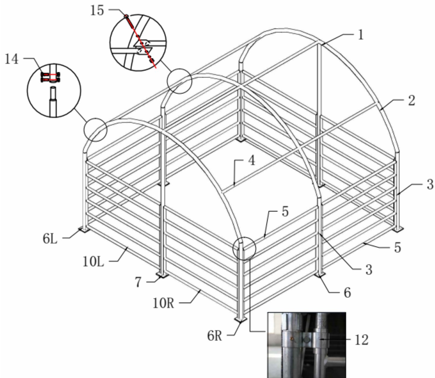
Kuva 1: Teräsrunko
