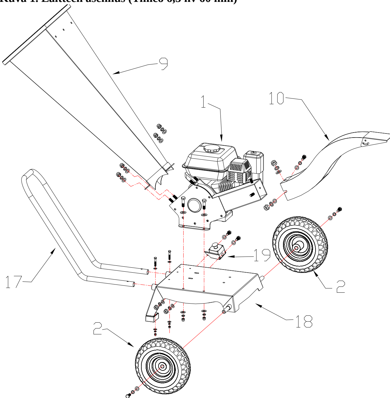
Kuva 1. Laitteen asennus (Timco 6,5 hv 60 mm)
